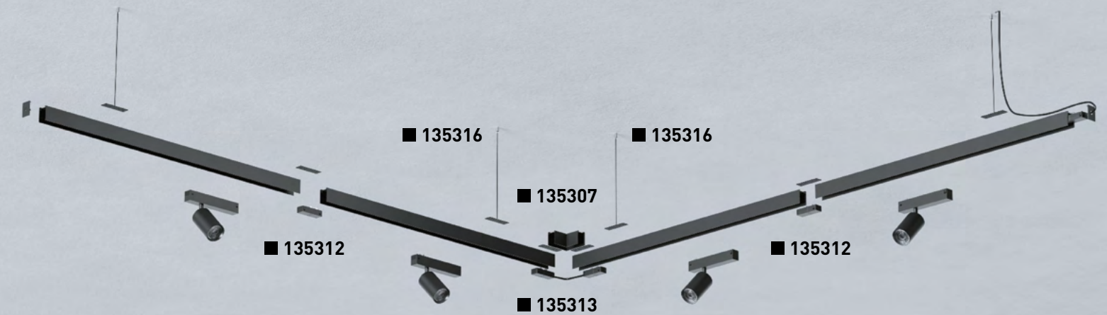
СХЕМА СБОРА
