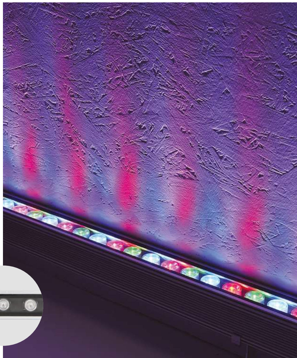
арт. 32257 (12 Вт, длина 500 мм) LL-892 арт. 32258 (18 Вт, длина 1000 мм) арт. 32259 (36 Вт, длина 1000 мм)
