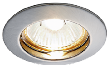
863A SN сатин, никель MR16 GU5.3 Ø78*4mm Ø65mm
