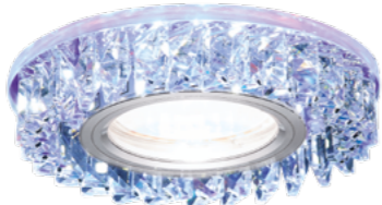
S255 PR хром/перламутровый MR16 GU5.3 3W 4200K Ø95*33mm Ø65mm
