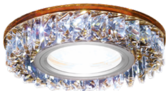
S255 BR хром/коричневый MR16 GU5.3 3W 4200K Ø95*33mm Ø65mm
