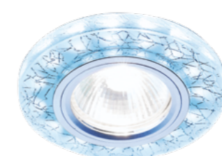
S226 W/CH/C хром белый, серебро MR16 GU5.3 3W 6400K Ø90*22mm Ø65mm
