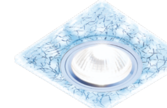
S227 W/CH/C хром белый, серебро MR16 GU5.3 3W 6400K 90*90*22mm Ø60*60mm
