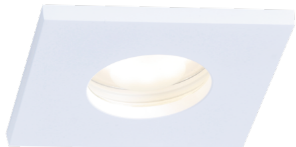
TN106 белый MR16 GU5.3 85x85x30 Ø70 IP44
