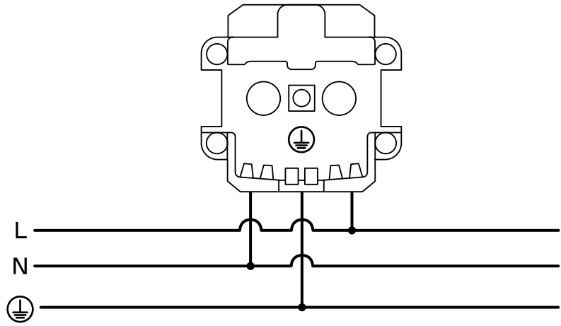
РОЗЕТКИ ЭЛЕКТРИЧЕСКИЕ ↗
