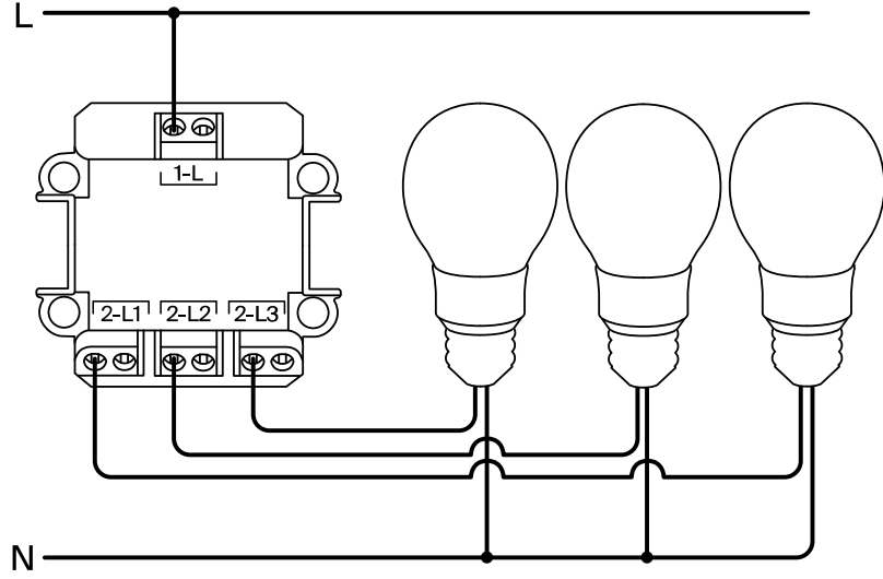
ВЫКЛЮЧАТЕЛЬ ТРЕХКЛАВИШНЫЙ ↘
