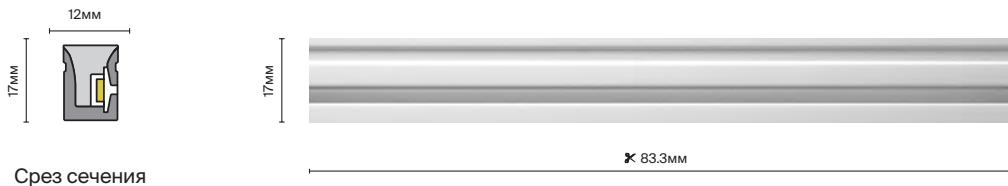
Срез сечения
